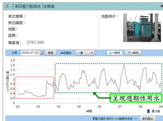
圖 5.2 一週壓力趨勢圖觀測
