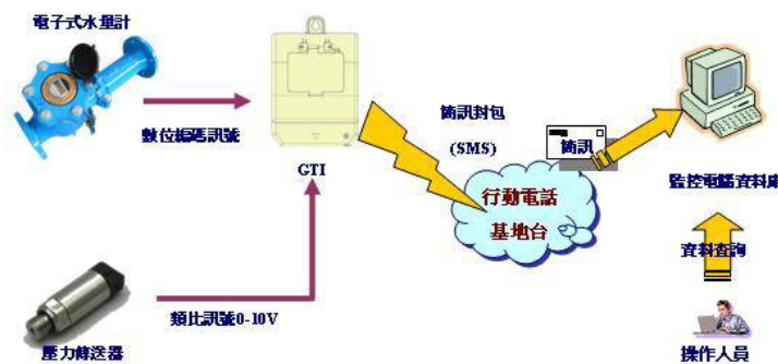
圖 4.8 新莊壓力監測系統架構圖
